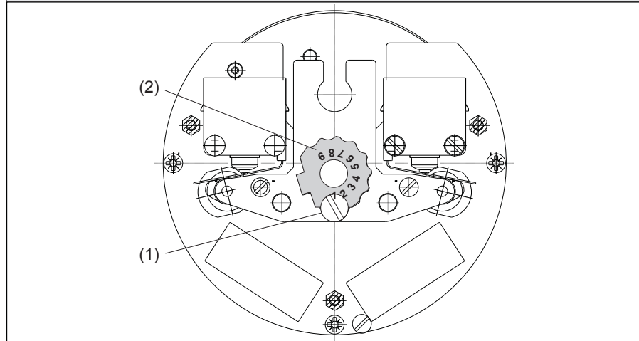
Рис 43: Понижающая передача
