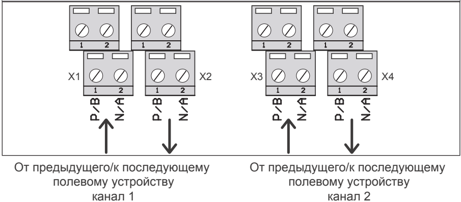
Рис 21: Плата подключения (для дублирования)
